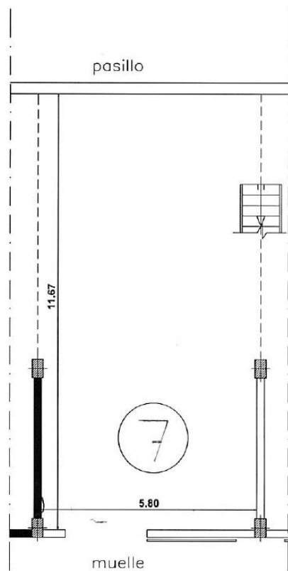
PLANTA BAJA
