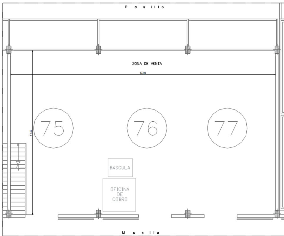
PLANTA BAJA
