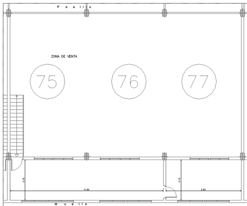
PLANTA ALTA
