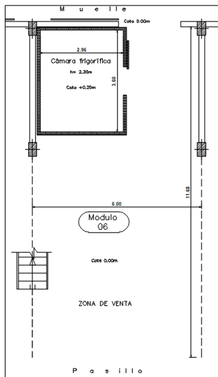
PLANTA BAJA
