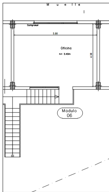
PLANTA ALTA
