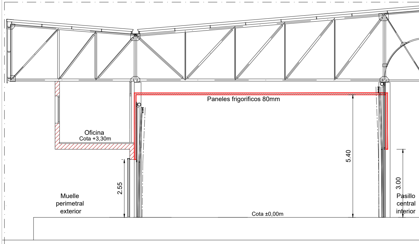
SECCION LONGITUDINAL
